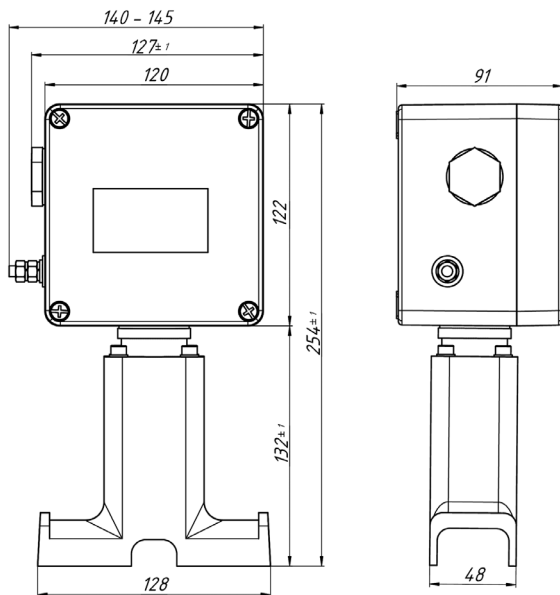
Габаритные размеры
